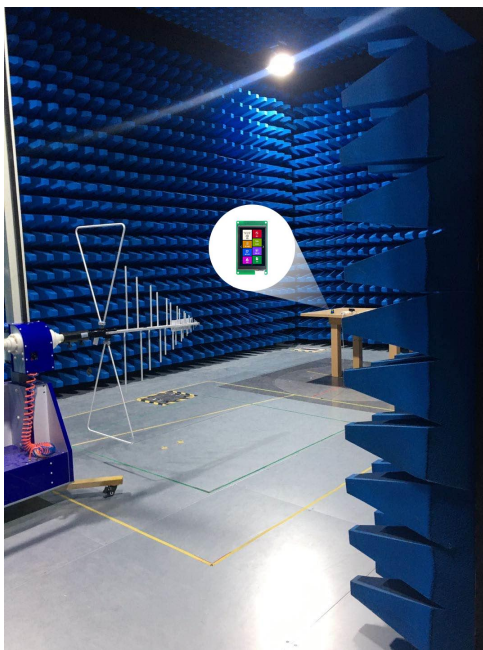
图 5-5 辐射测试图
