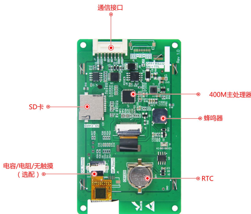
图 1-4 硬件配置图
